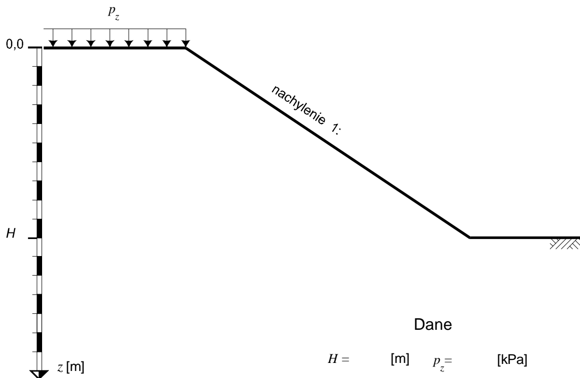
Przekrój skarpy
