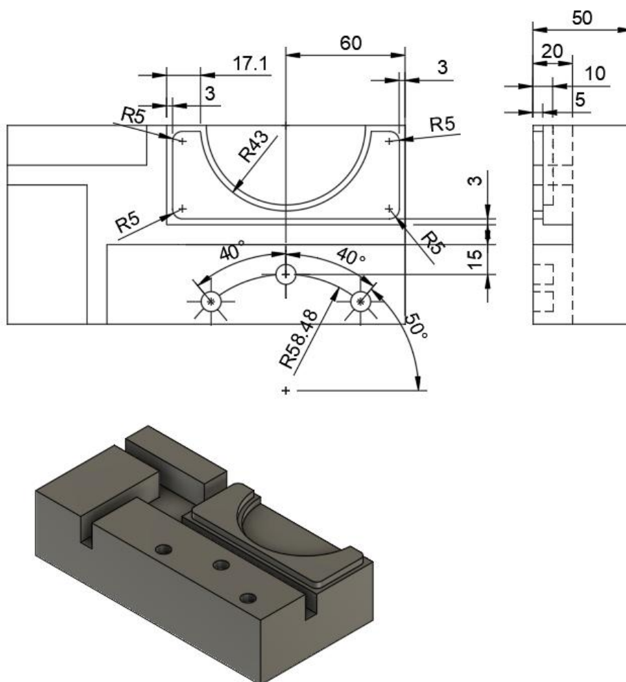
Rys.1. Detal
